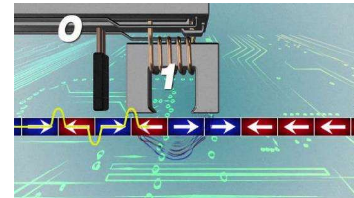
面内磁気記録方式
